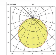
עקומות פוטומטריות:
